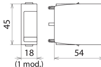
Beépítési méretek DG MOD ACI 275
